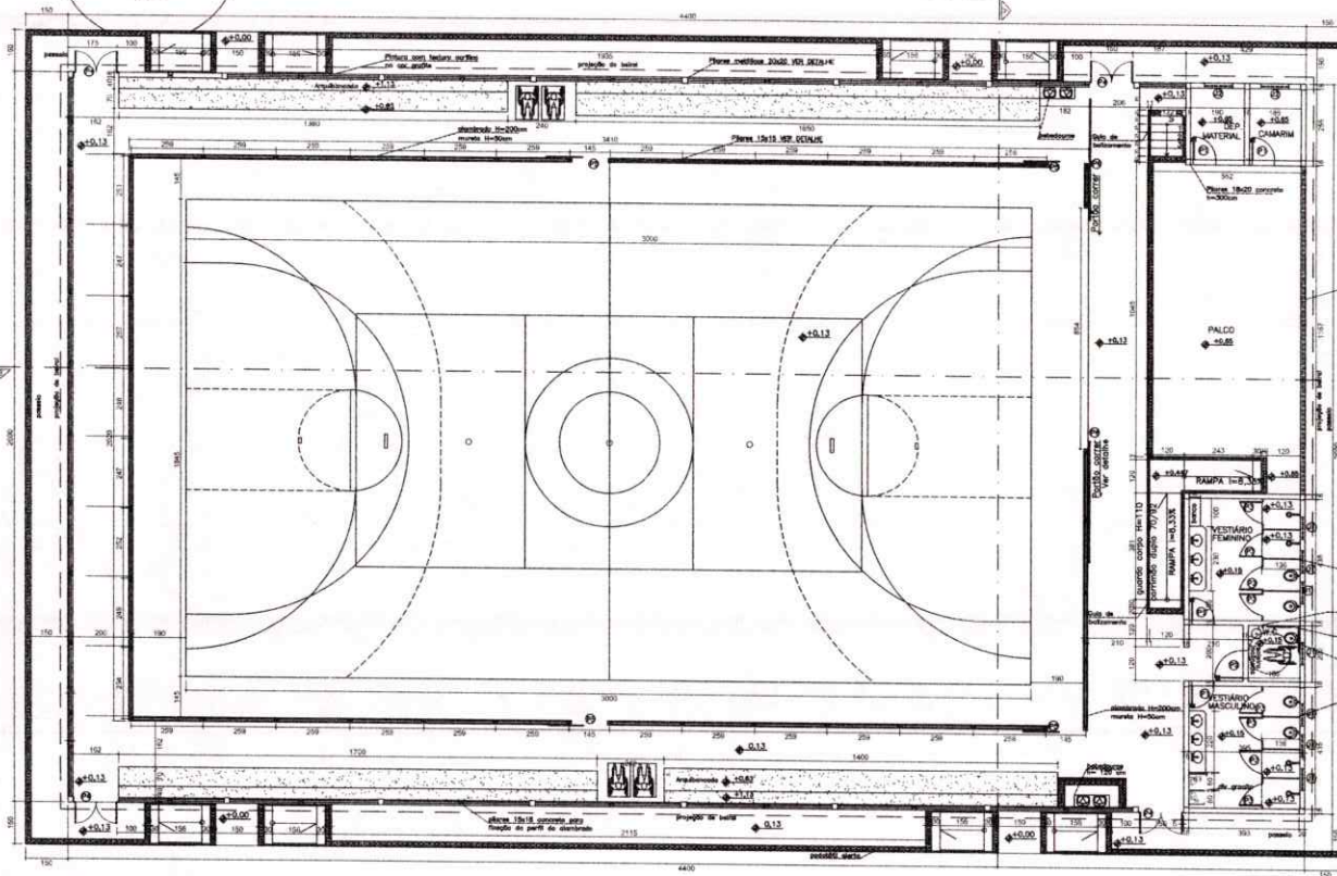
PLANTA QUADRA COBERTA S= 1144,00m 2 escala 1/100
